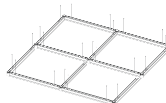
Conector en "X"
